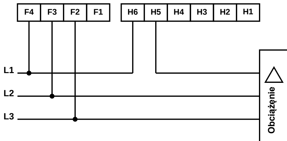
[ 3W BAL ] : 3-przewodowa symetryczna bez zera
