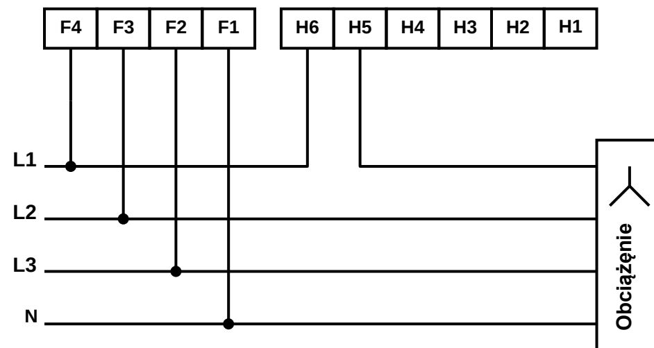
[ 4W BAL ] : 3-przewodowa symetryczna z zerem
