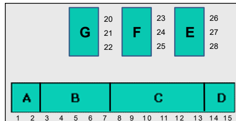
Schéma de l'emplacement des borniers (vue du boîtier en face arrière)
